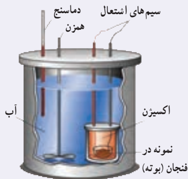
شکل ۴-۲۲ اجزای یک گرماسنج بمبی
