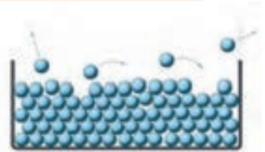
شکل ۴-۲۵ در حین تبخیر سطحی، مولکول‌های پر انرژی‌تر از سطح مایع می‌گریزند.
