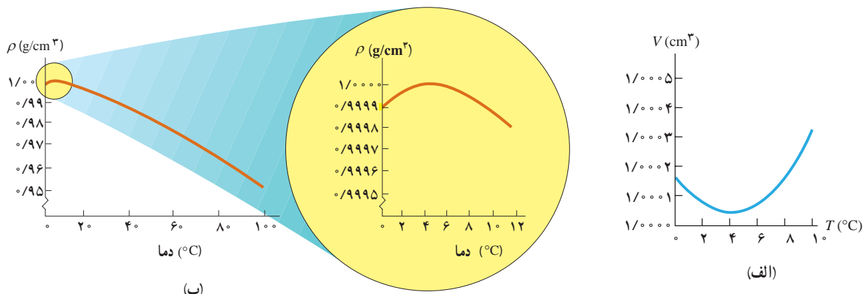
شکل ۴-۱۴ (الف) تغییرات حجم یک گرم آب (شیرین) با دما، (ب) تغییرات چگالی آب (شیرین) با دما
